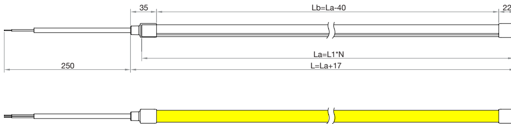
Alimentazione assiale / Axial Powercap
