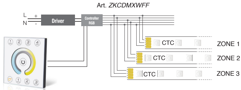
Esempio di connessione con pannello: Example of connection to CTC panel: Art. ZKTPC-CTC
